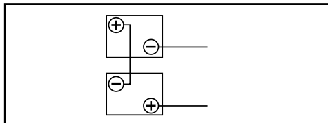
Foto 12 Connessione delle batterie
