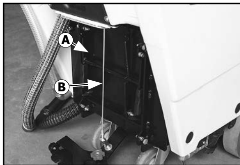
Foto 9 A) Sportello di accesso al vano batterie (optional) B) Cavo di sollevamento del tergilavaggio
